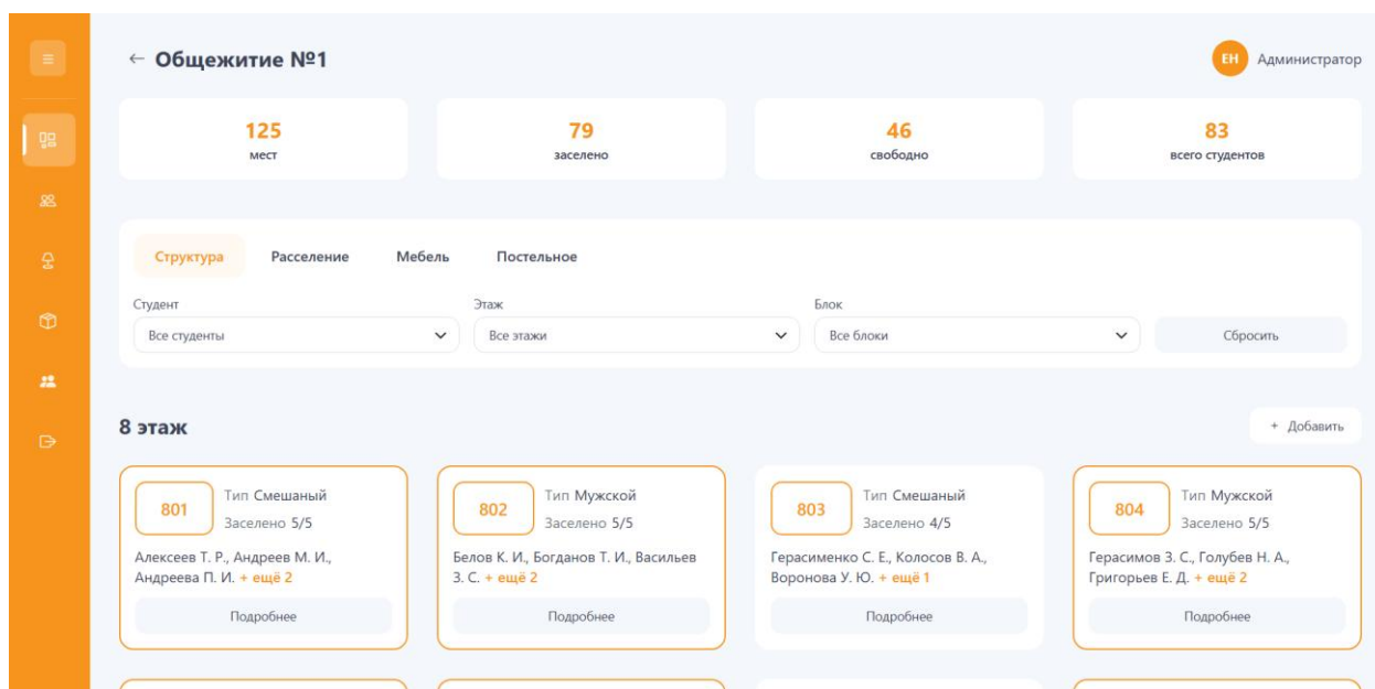
Рисунок 17 – УНФО. Вид вкладки «Структура»
